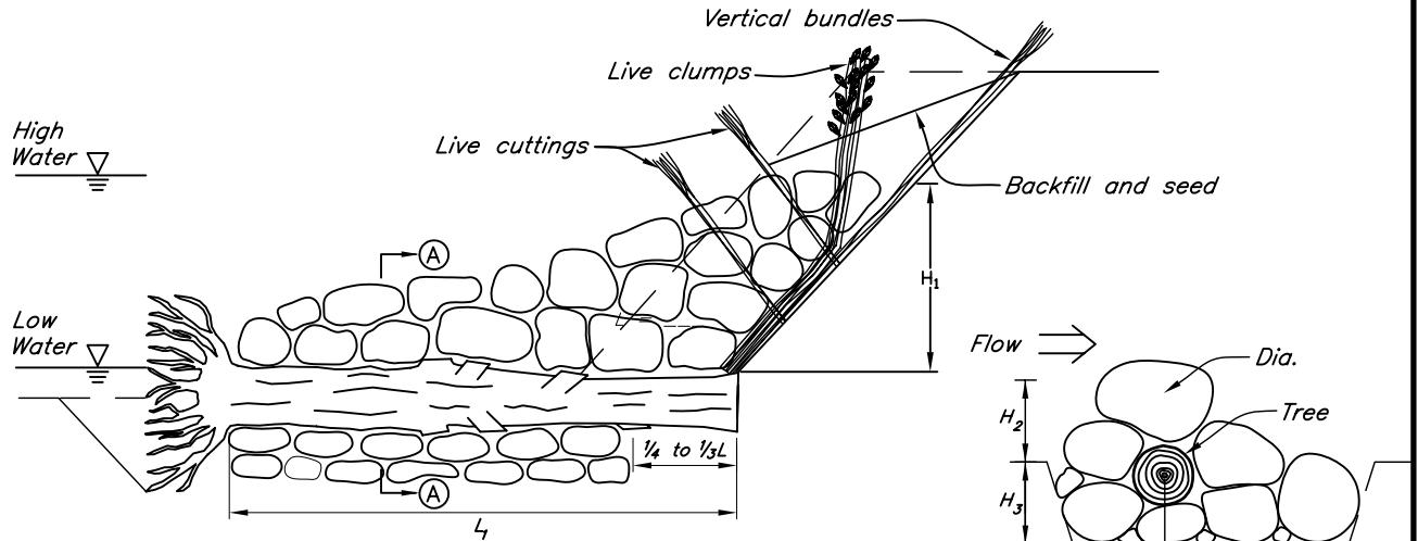
ROCK BARB WITH ROOT WAD (PROFILE) N.T.S.
